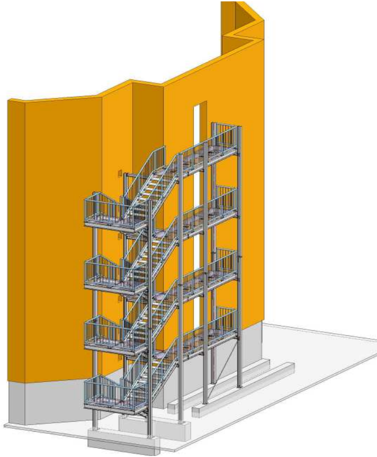
3D Zeichnung in HiCAD ( Planung von B&S Stenzel GmbH )
